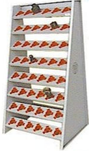
KOD NO. MT-05 Mors Tutucu Sehpa (48 Adet)
