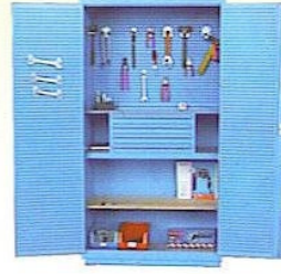
KOD NO. MD-01 4 Çekmeceli 190 x 100 x 50 cm.
